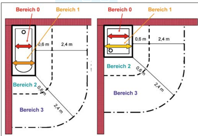
Schutzbereiche im Badezimmer.
