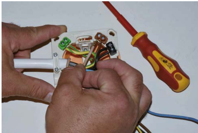
Anschluss der Herdanschlussleitung an der Herdanschlussdose.
